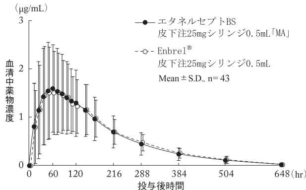
図1 エタネルセプトBS皮下注25mgシリンジ0.5mL「MA」及びEnbrel®皮下注25mgシリンジ0.5mL単回投与後の血清中薬物濃度推移
