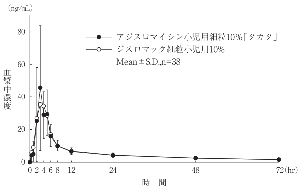
図 16-1 血漿中濃度（細粒 10%）
