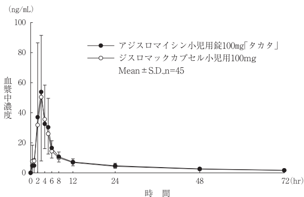
図 16-2 血漿中濃度（錠 100mg）
