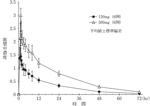
図1 本剤単回点滴静注後の血漿中ラスクフロキサシン濃度推移 ( \mu\text{g/mL} )
