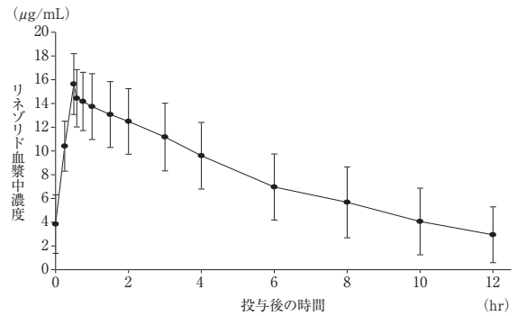
図1 リネゾリド625mgを1日2回12時間ごとに反復静脈内持続投与した後の定常状態における血漿中濃度推移(Mean ± S.D.、外国人、n=6)
